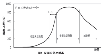
図2 区画火災の成長
